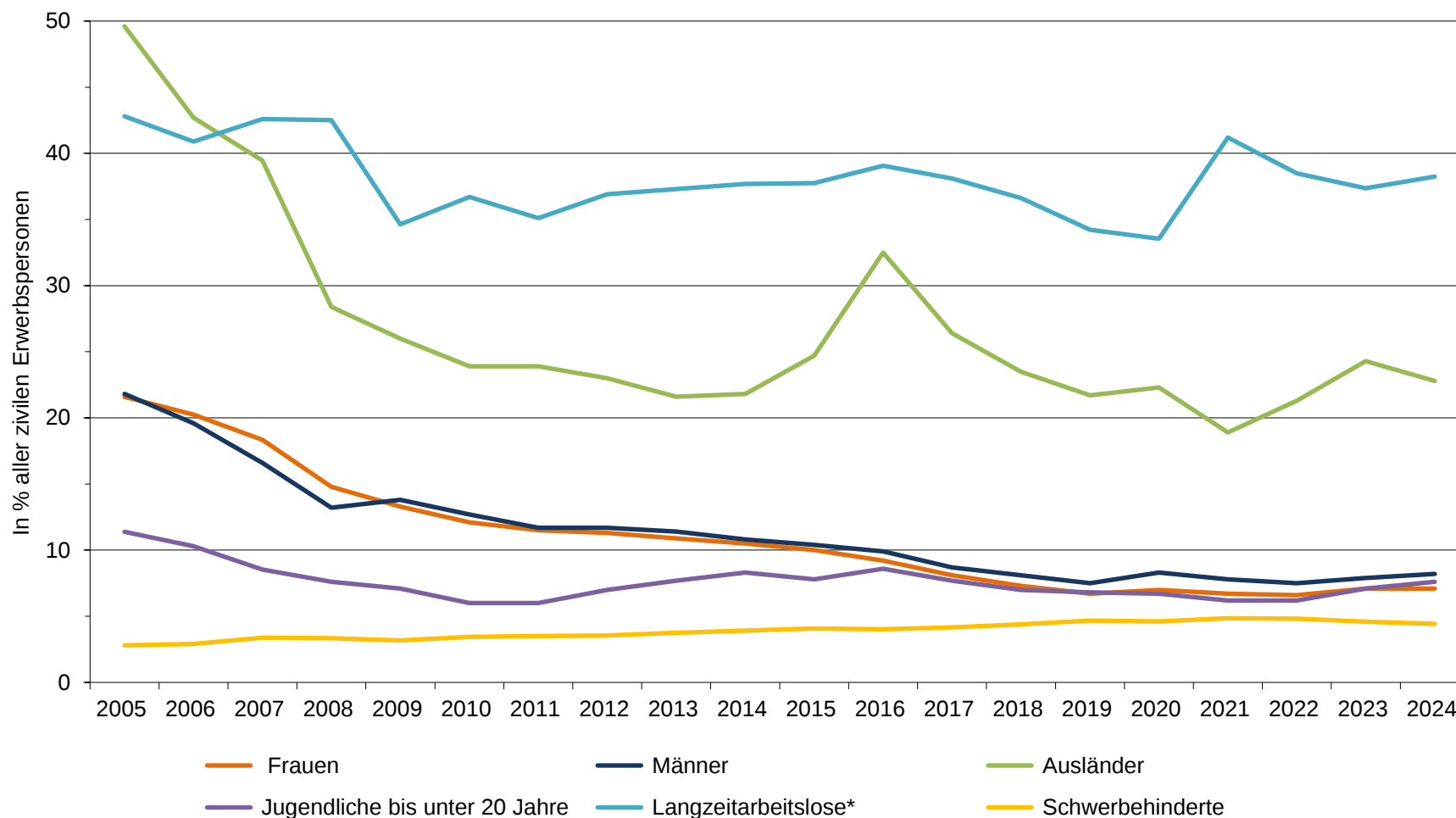
2.20 (K): Arbeitslosenquote (Jahresdurchschnitt in % aller zivilen Erwerbspersonen), nach Geschlecht, Sachsen-Anhalt, 2005–2024
